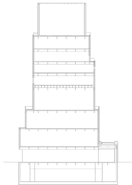
剖面圖
