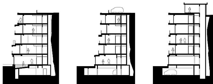
懸崖酒店剖面圖
